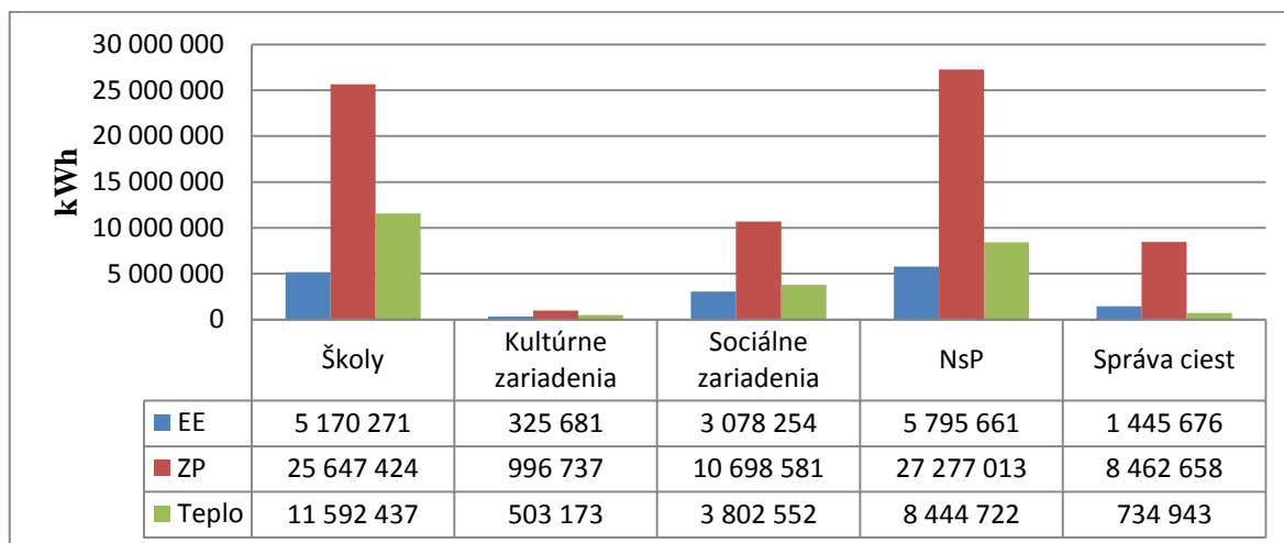
Obrázok 27: Spotreba podľa účelu využitia jednotlivých objektov TSK (kWh)
