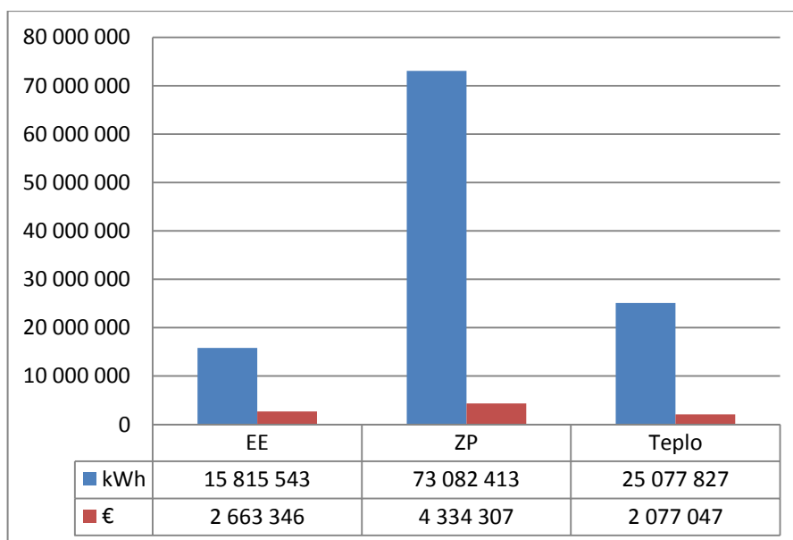
Obrázok 50: Podiel zdrojov v kWh a vo finančnom vyjadrení pre všetky objekty TSK
