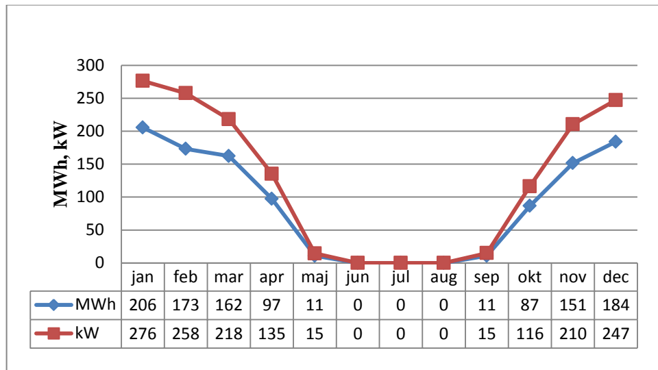
Obrázok 25: Priebeh ročnej spotreby tepla Q a výkonu P
