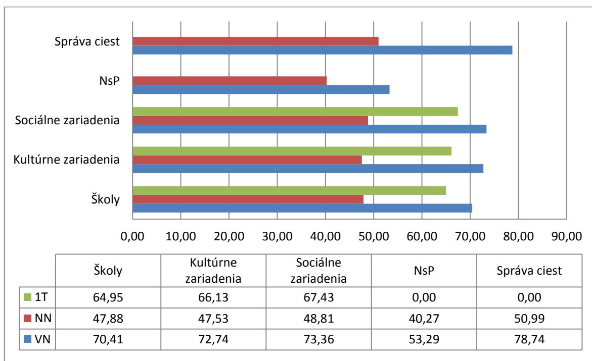
Obrázok 60: Prehľad priemerných cien elektrickej energie v referenčnom roku podľa účelu zariadení
