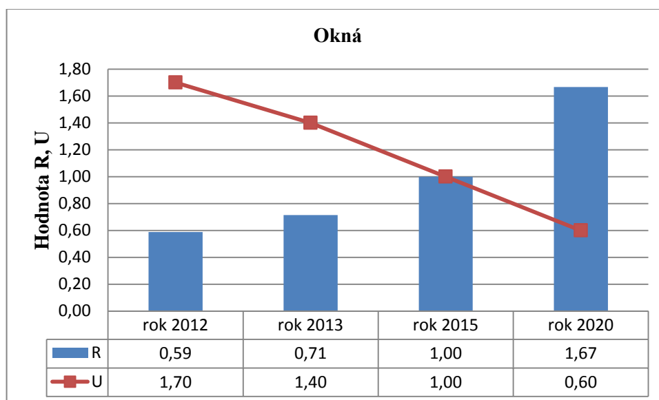
Obrázok 46: Okná R a U
