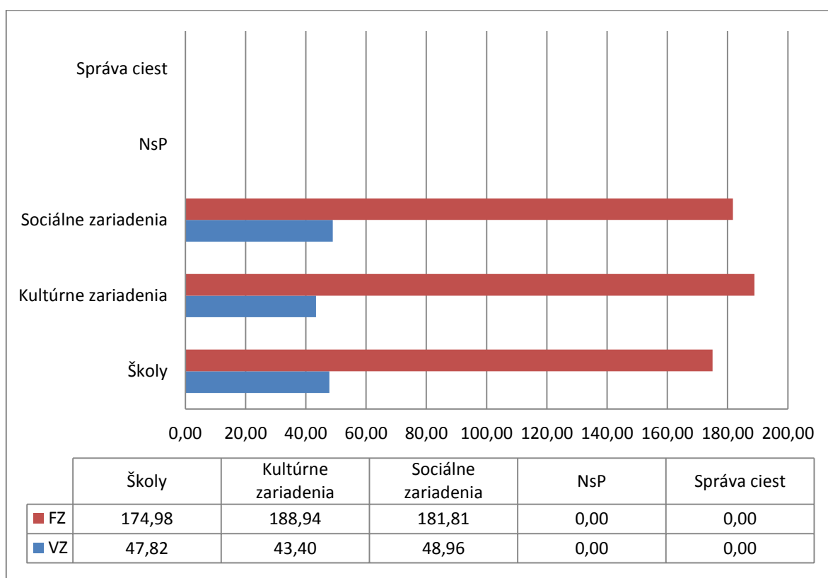
Obrázok 64: Prehľad priemerných cien tepla v referenčnom roku podľa účelu zariadení
