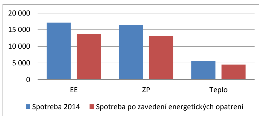
Obrázok 66: Porovnanie produkcie CO 2 (t)
