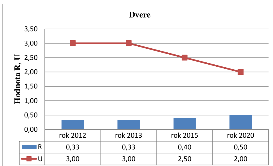
Obrázok 47: Dvere R a U
